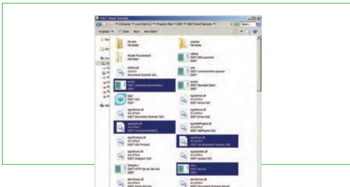
شکل ۳-۶ پنجره Computer
