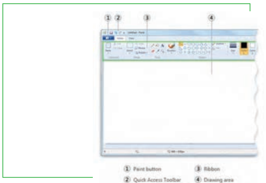
شکل ۲۳-۳ نرم‌افزار Paint
